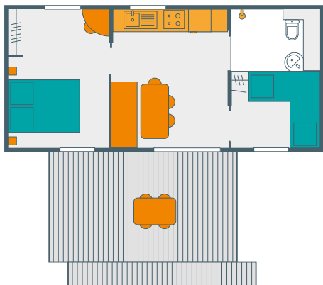
MOBIL-HOME PREMIUM 2 CHAMBRES | PMR 4 PERS. | 32 M 2 | FAÇADE ET TERRASSE BOIS
