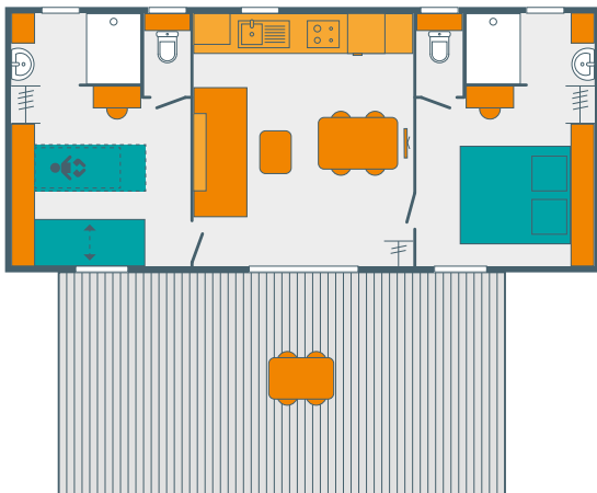
MOBIL-HOME PRESTIGE 2 CHAMBRES 2 SDB 4 PERS. | 35 M 2 | FAÇADE ET TERRASSE BOIS
